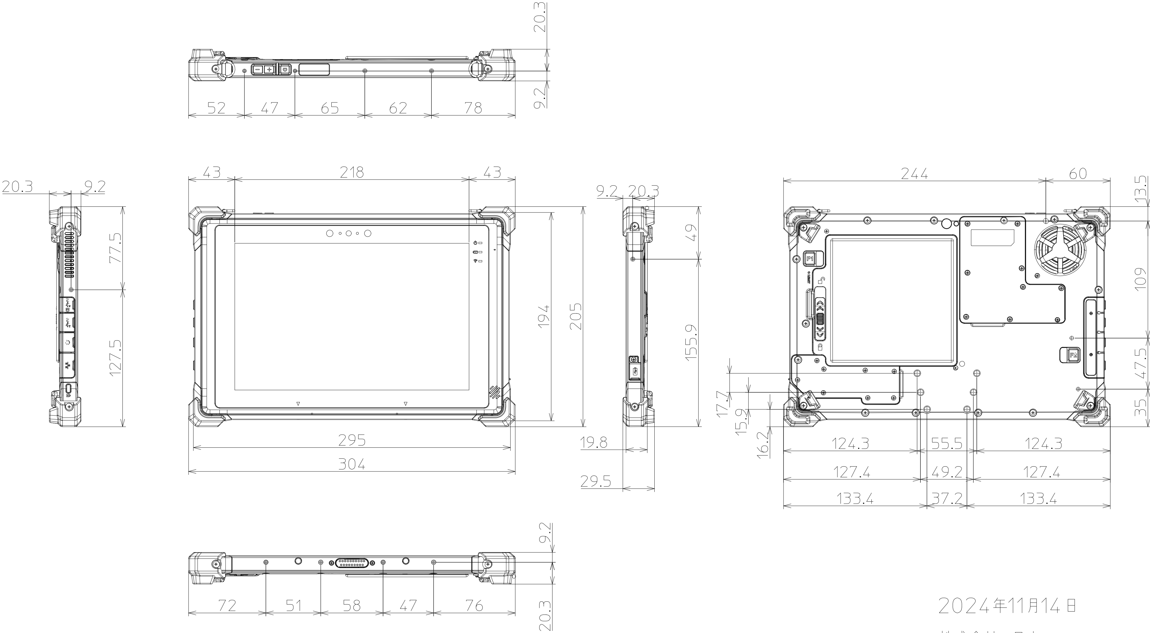
堅牢タブレット（RG1シリーズ）外観図（ご参考）
